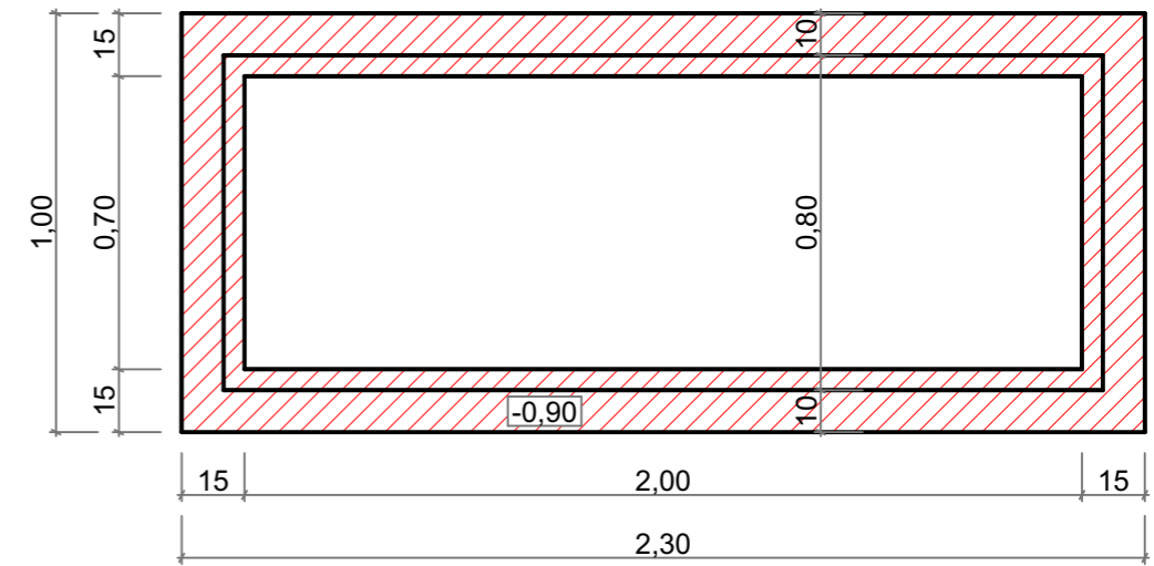
PLAN FUNDAȚIE
