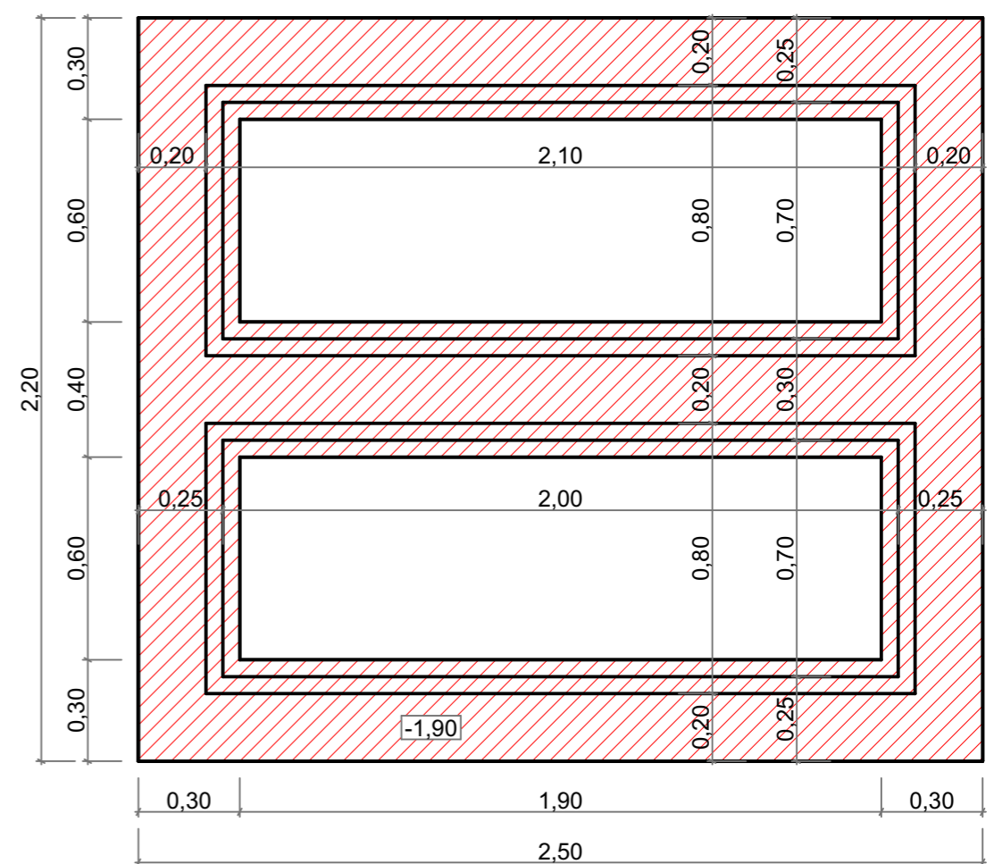
PLAN FUNDAȚIE
