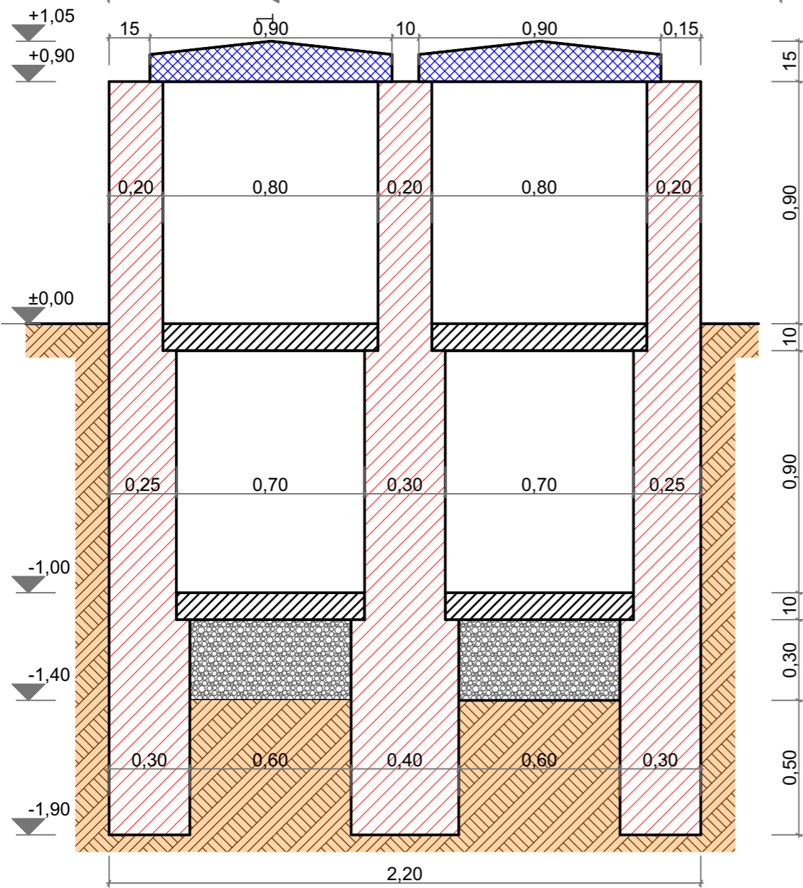
SECȚIUNE 1-1
