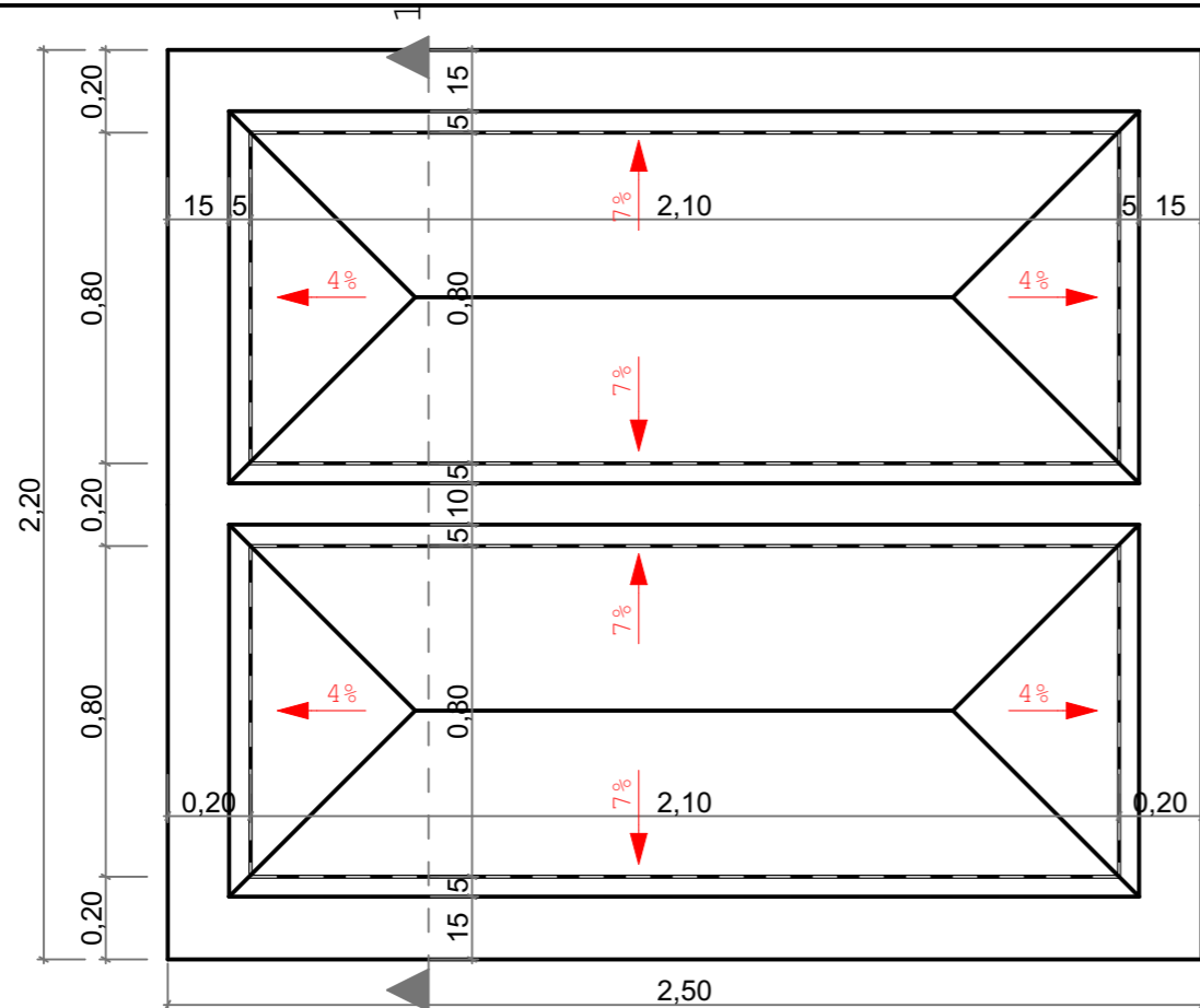
PLAN CRIPTĂ
