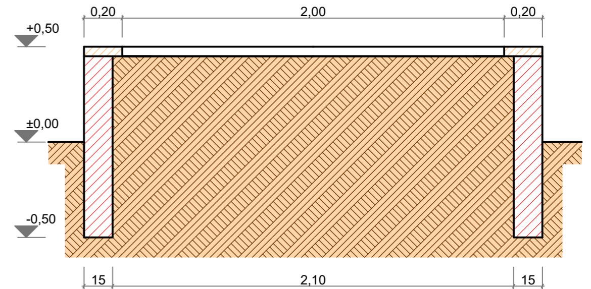
SECȚIUNE 1-1
