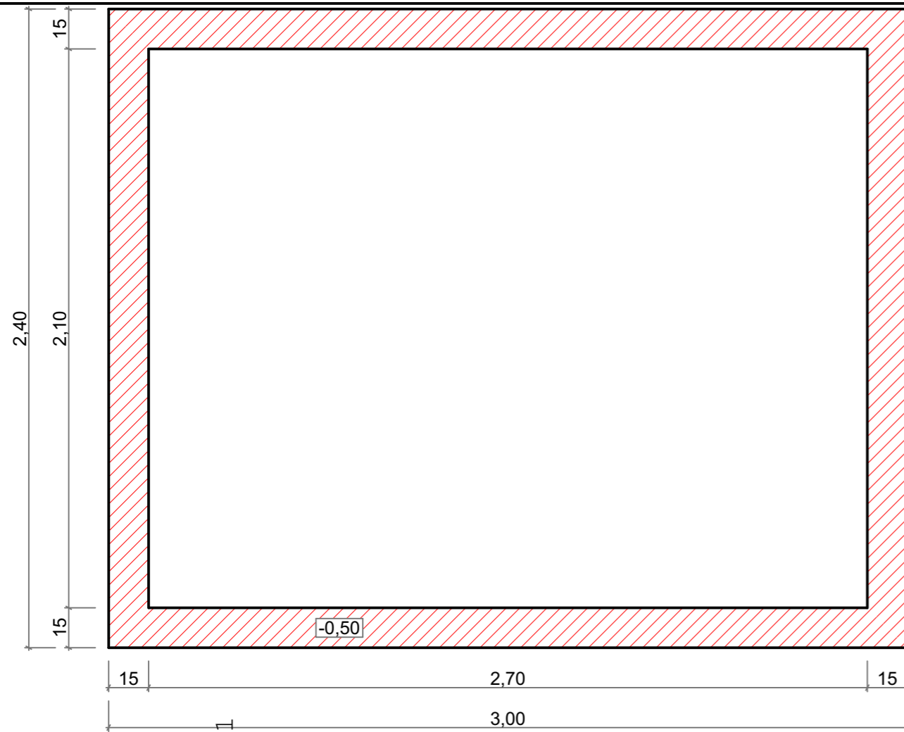
PLAN FUNDAȚIE
