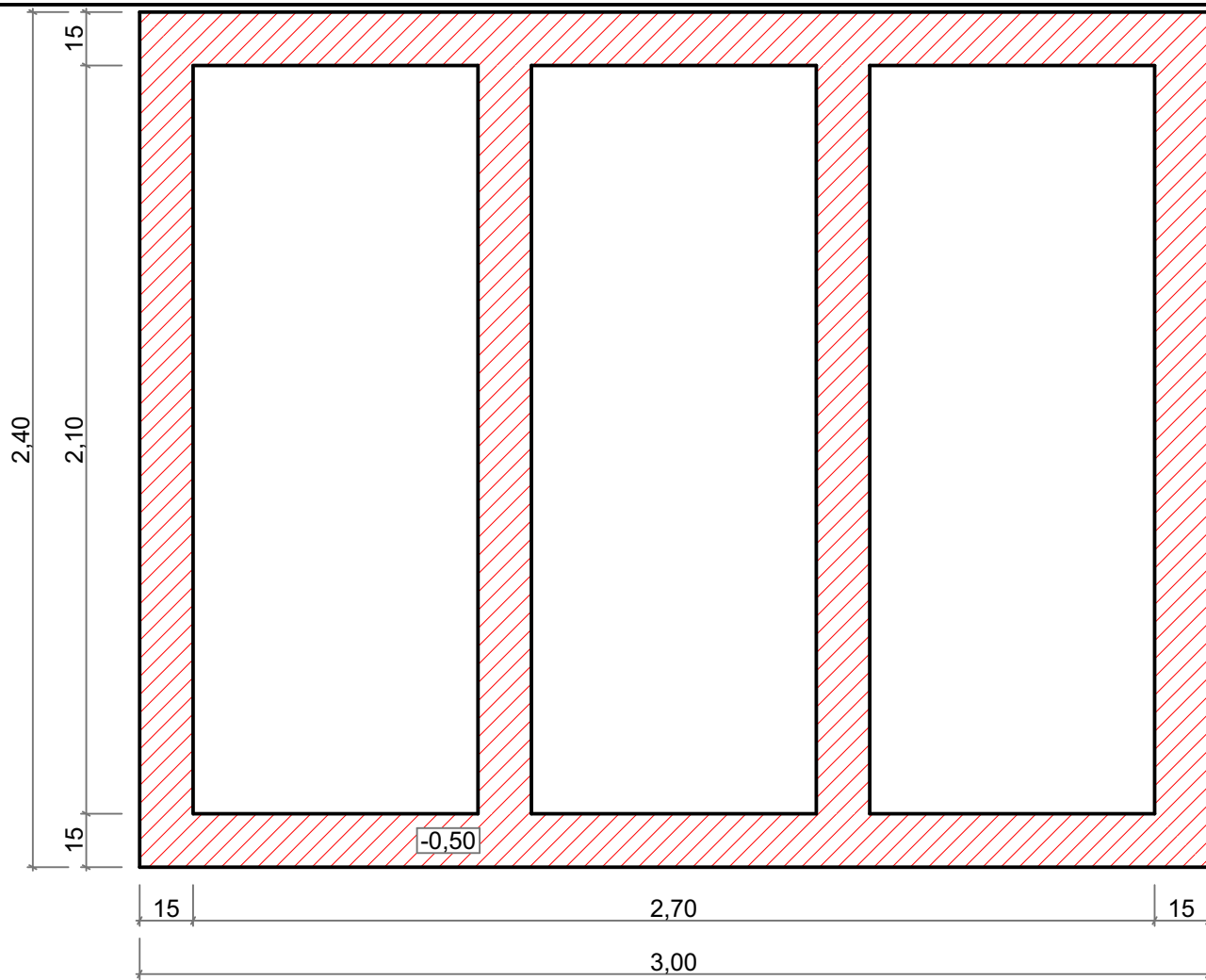
PLAN FUNDAȚIE
