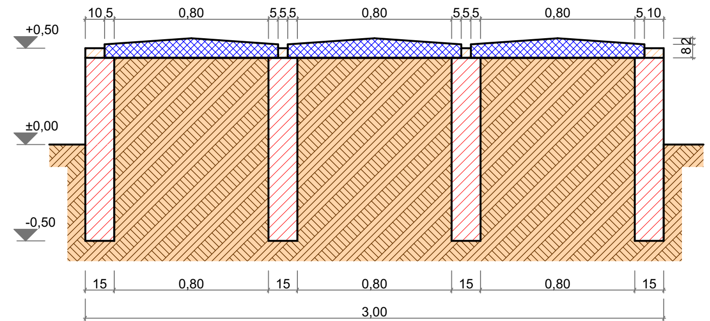
SECȚIUNE 1-1
