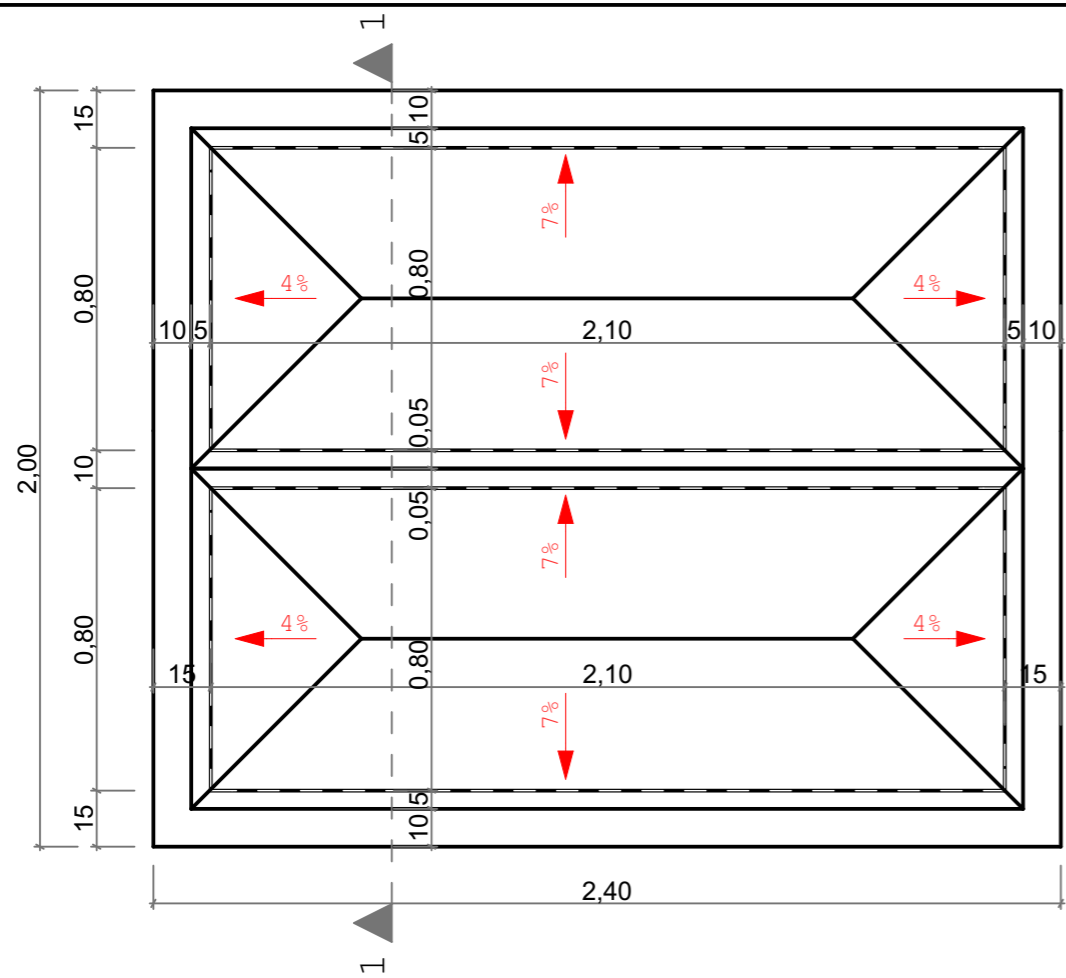
PLAN CRIPTĂ
