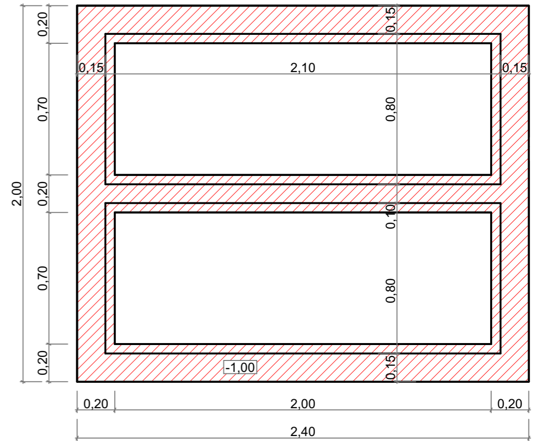
PLAN FUNDAȚIE
